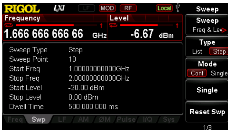
Рисунок 10. Интерфейс настройки параметров выходного сигнала радиочастотной развертки
